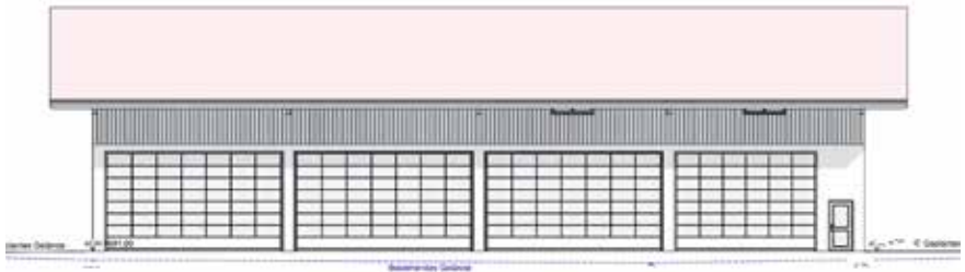
Ansicht Süd- Ost
